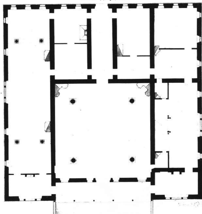
План дворца Г.А. Потемкина
