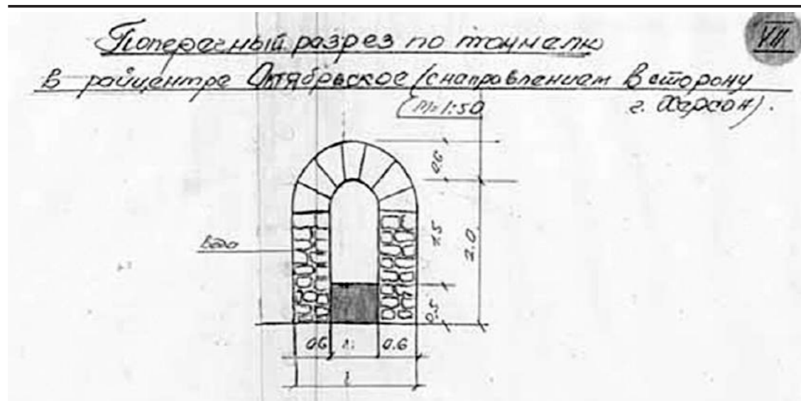
Рисунок тоннеля в Октябрьском из доклада инженера Алексева
