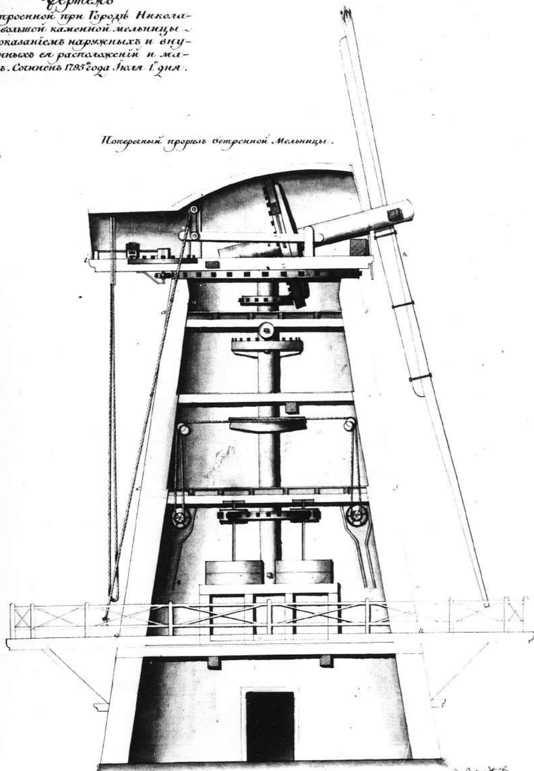
Чертеж ветряной мельницы
