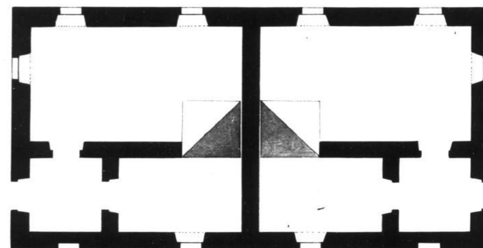
Чертеж дома для мастеров-гутников
